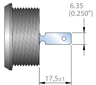
'fast-on' F2
