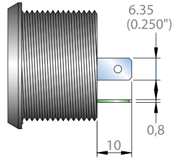
'fast-on' F2
